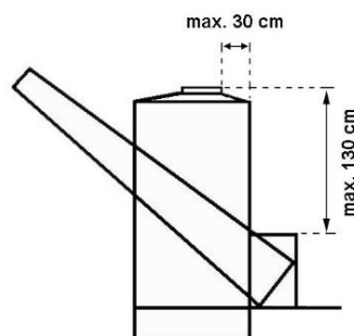
Maximale Abstände für die Erreichbarkeit der Einfüllöffnung
