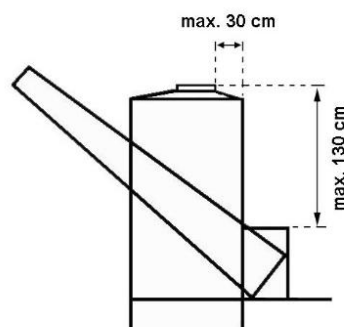
Maximale Abstände für die Erreichbarkeit der Einfüllöffnung
